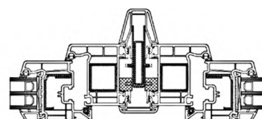
в) Торцевое соединение коробок с использованием фасадного соединителя (с возможностью компенсации температурных деформаций)
