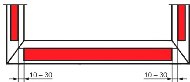
Рисунок 9 — Пример установки усиленных вкладышей в профилях ПВХ
