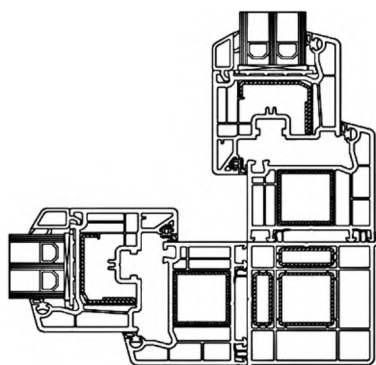
г) Угловое соединение коробок с использованием углового 90° усилителя
