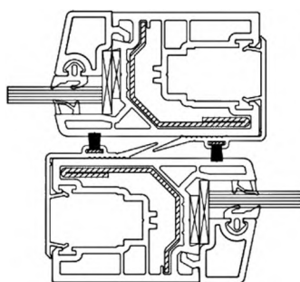
л) Притвор балконного остекления с раздвижным открыванием створок
