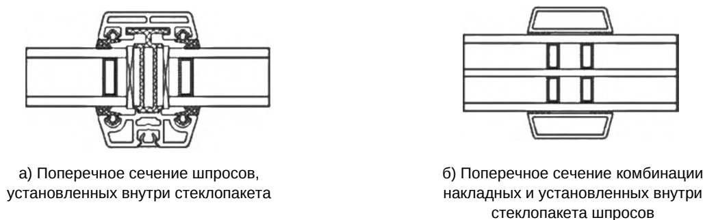
Рисунок 6 — Варианты установки декоративных раскладок
