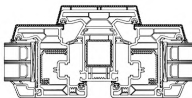
б) Импостный притвор с двумя открывающимися створками для оконных блоков с декоративными алюминиевыми накладками
