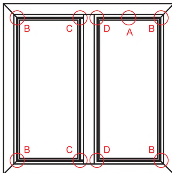
Рисунок Г.1 — Схемы установки уплотняющих прокладок в створке и раме с импостом оконного блока из профилей ПВХ
