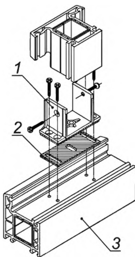
1 — колодка; 2 — уплотнительная пластинка; 3 — рама, импост или створка
