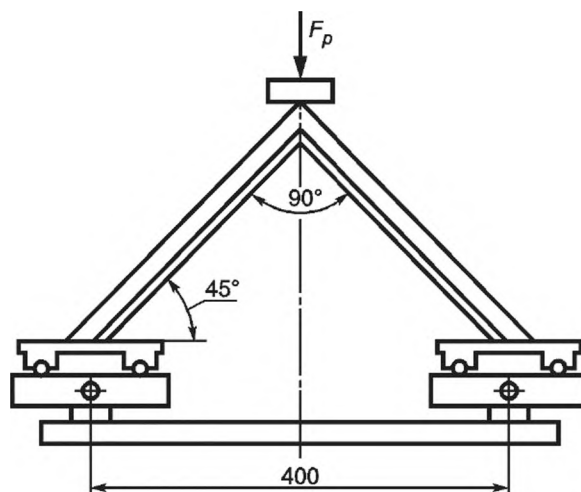
Рисунок 11 — Схема Б приложения разрушающей нагрузки F_p при определении прочности угловых соединений
