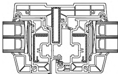
ж) Штульповый притвор для оконных блоков со скрытыми створками
