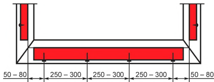
а) Схема крепления усиленных вкладышей в профилях ПВХ белого цвета
