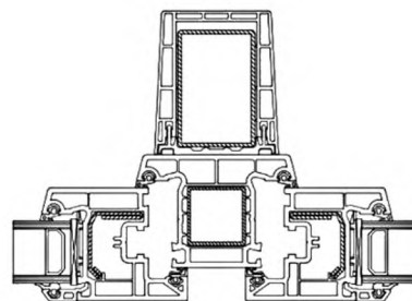
к) Импостный притвор с внешним усилителем
