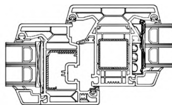
в) Импостный притвор с одной открывающейся створкой
