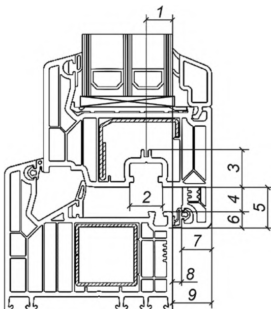
Рисунок А.1 — Основные элементы оконных блоков из профилей ПВХ
