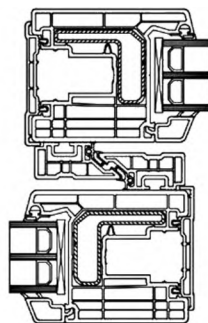
и) Притвор систем панорамного остекления с подъемно-раздвижными створками
