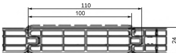
Рисунок 7 — Пример многокамерного профиля ПВХ для изготовления филенок
