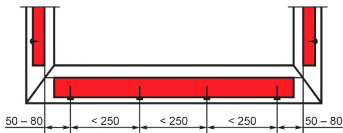
б) Схема крепления усиленных вкладышей в цветных профилях ПВХ
