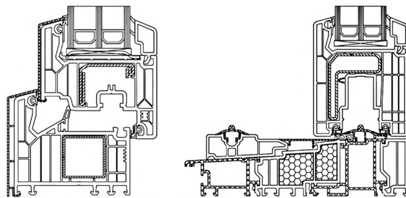
к) Оконный блок из многокамерных профилей с декоративными алюминиевыми накладками
