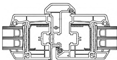
д) Штапеловый притвор
