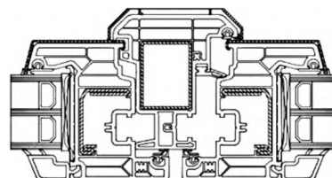
е) Штапеловый притвор для оконных блоков с декоративными алюминиевыми накладками
