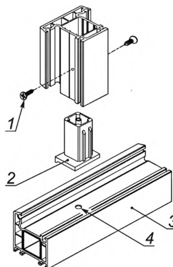
1 — шурупы; 2 — соединитель импоста; 3 — рама; 4 — отверстие
