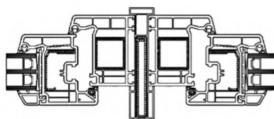
б) Торцевое соединение коробок с использованием усиленного соединителя (без возможности компенсации температурных деформаций)
