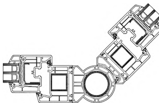
д) Угловое соединение коробок с использованием углового универсального усилителя
