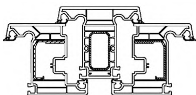
а) Импостный притвор с двумя открывающимися створками
