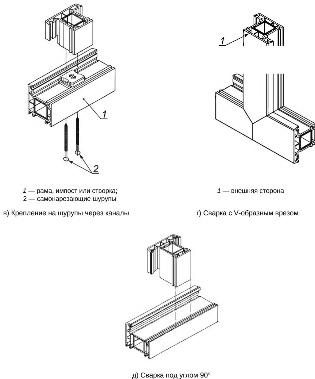
Рисунок 4 — Примеры крепления импостов
