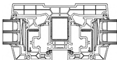
г) Импостный притвор с двумя открывающимися створками для оконных блоков со скрытыми створками
