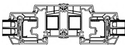
а) Торцевое соединение коробок с использованием мини-соединителей
